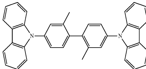
CDBP
