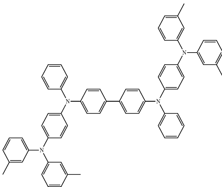
DNTPD
